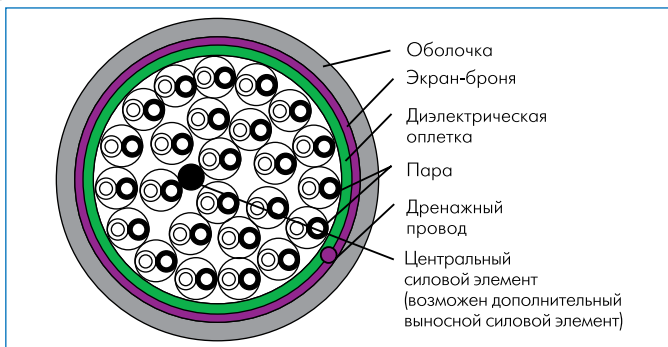
Рис. 1 Конструкция витой 25-парной FTP категории 5e
