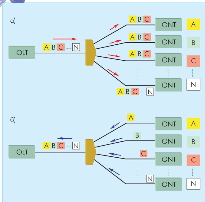
Рис. 1 Прямой поток (а) и обратный поток (б)
