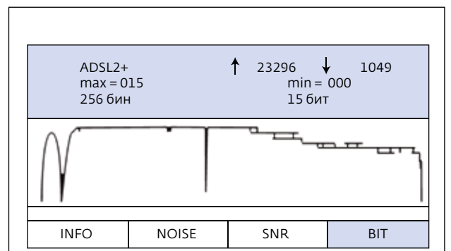
Рис.3. Побитовая характеристика скорости BitRate
