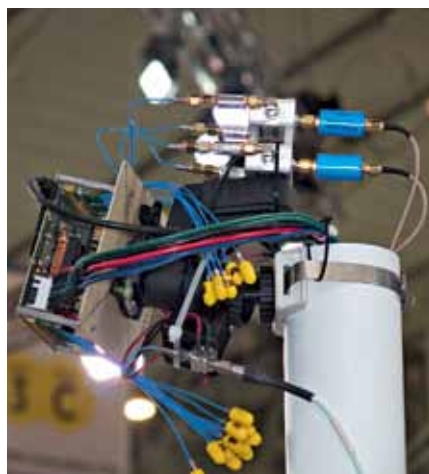
Прототип базовой станции миллиметрового диапазона
