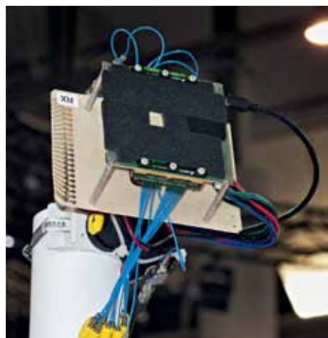
Прототип базовой станции миллиметрового диапазона
